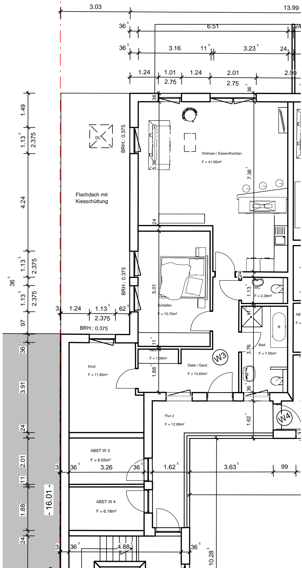
OBERGESCHOSS - Wohnung Nr. 3 M. 1:100
