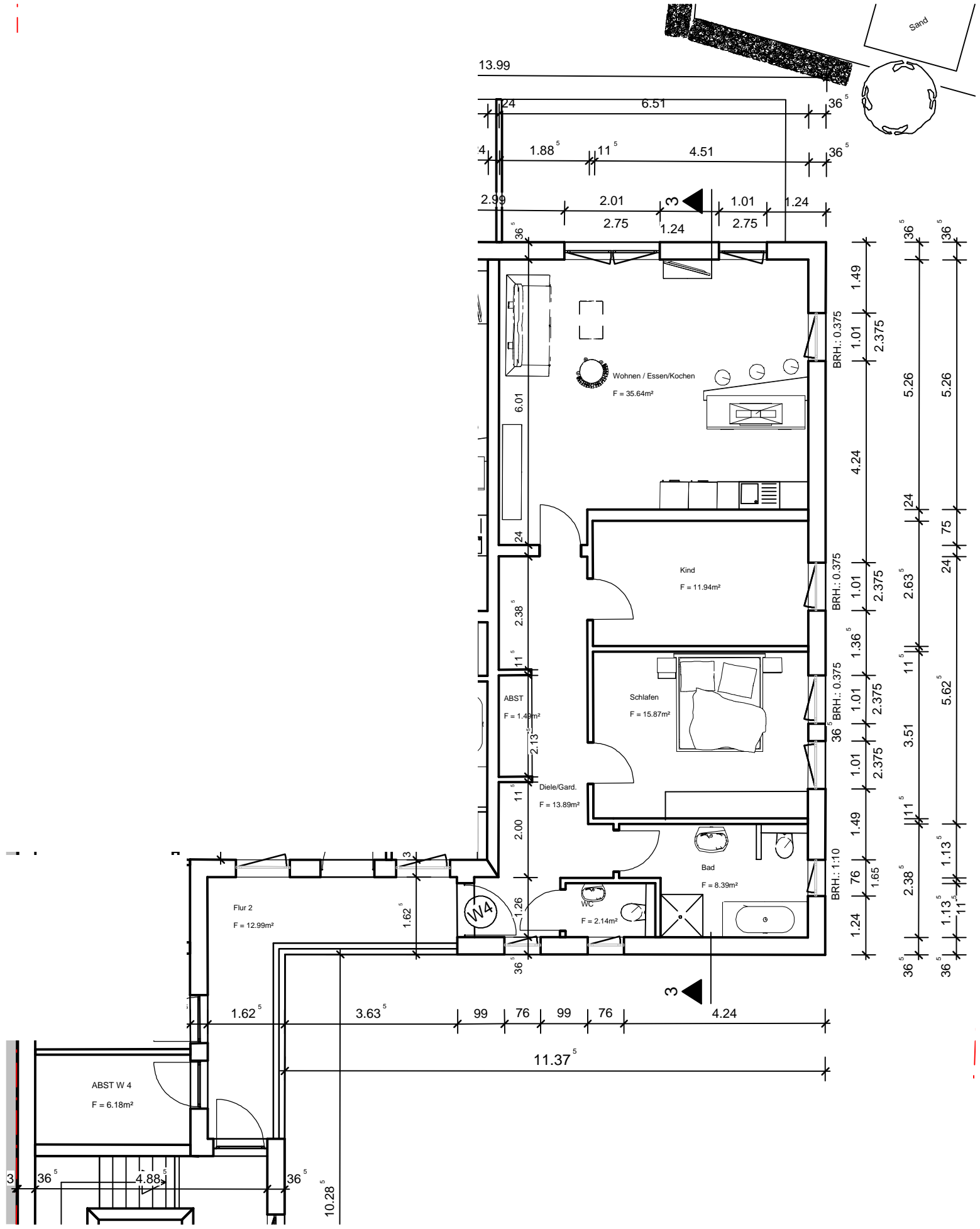
OBERGESCHOSS - Wohnung Nr. 4 M. 1:100
